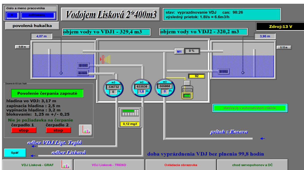
Obr. Dispečingový systém – Bloková schéma VDJ Lisková (2x400m3)
